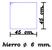
DETALLE - A Del Estribo: (Item 1)
