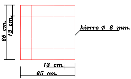
DETALLE - C PARRILLA p/Base De Pilar (Item 2)
