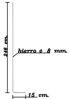
DETALLE - B (Item 2)
