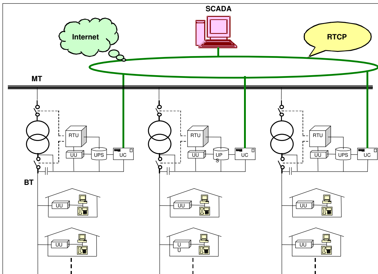
Fig. 2. Control de la red de energía y telecomunicaciones públicas integrados en un mismo sistema TRE
